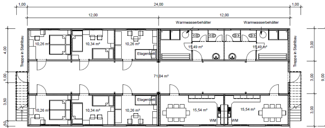
Grundriss EG
