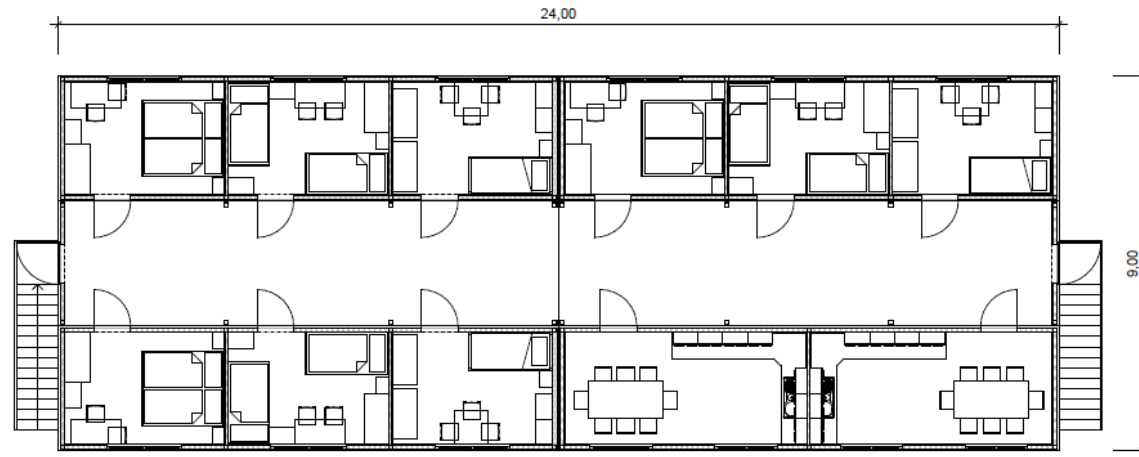
Grundriss OG
